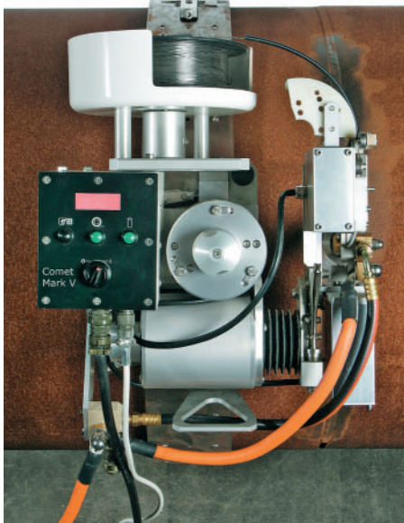
Orbitalschweißsystem Comet Mark V
